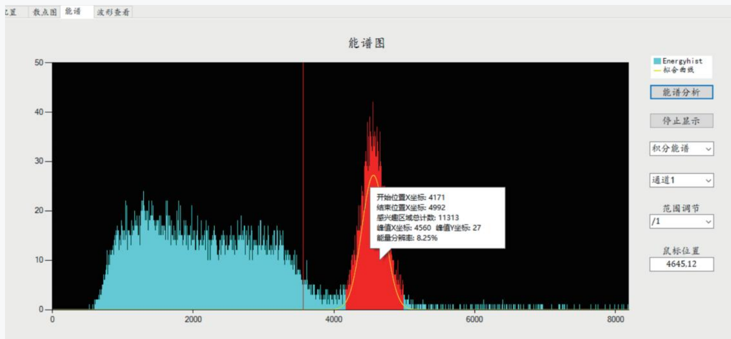
Cs-137采集60s能谱(紧贴晶体)
